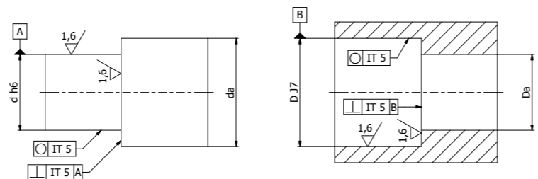
Housing PE
