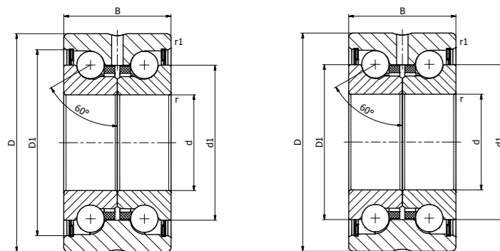
SEL/N...2RS / SEL/N...2RS.PE
